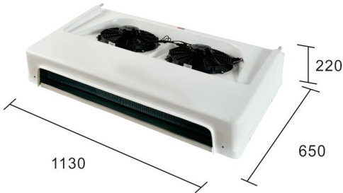
蒸发器 Evaporator
