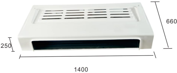
蒸发器 Evaporator
