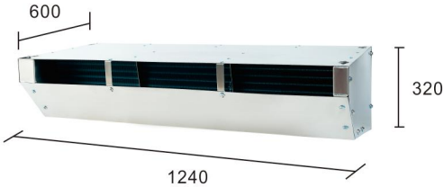
蒸发器 Evaporator
