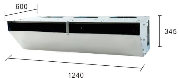
蒸发器 Evaporator
