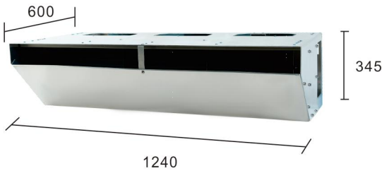
蒸发器 Evaporator
